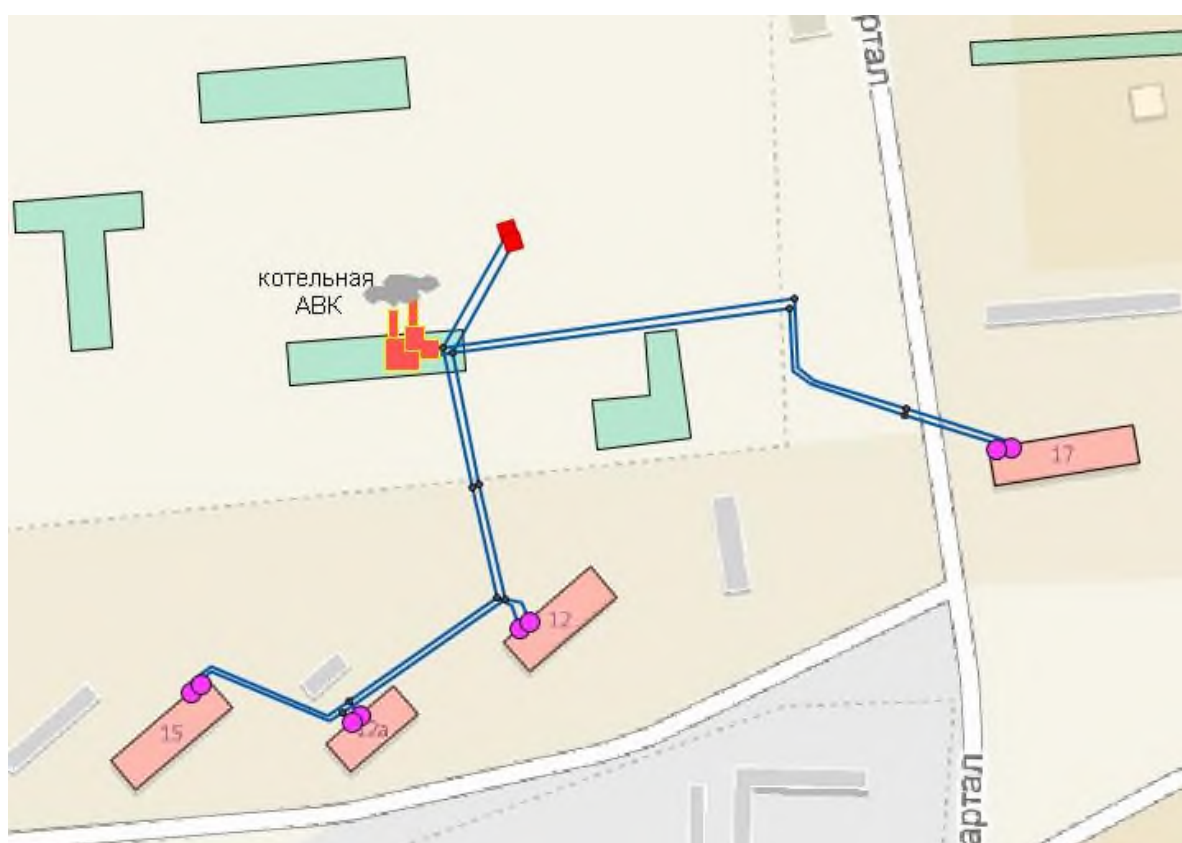
Рисунок 1.5 – Тепловые сети котельной Абаканской воспитательной колонии
