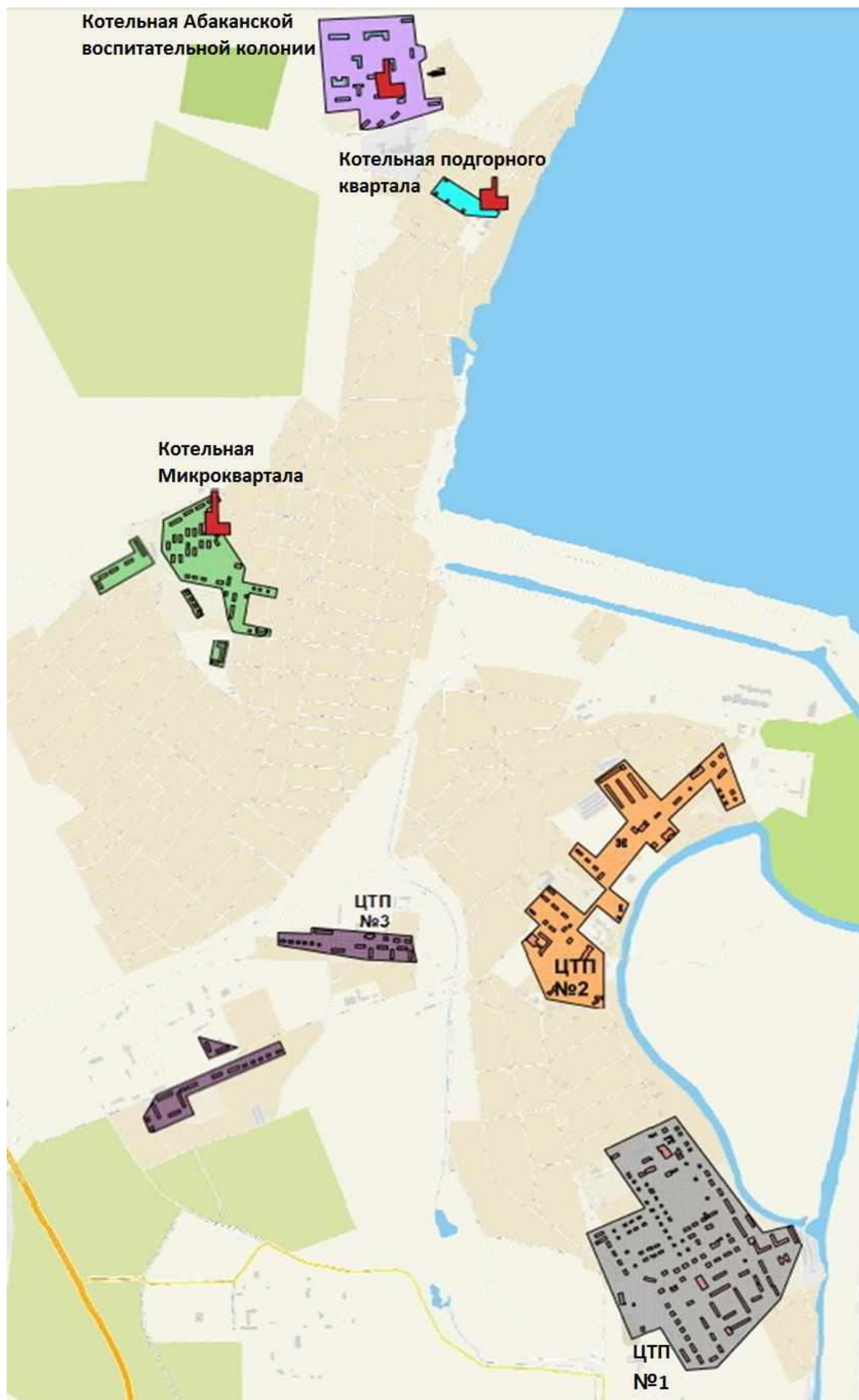
Рисунок 2.1 - Зоны действия систем теплоснабжения и источников тепловой энергии
