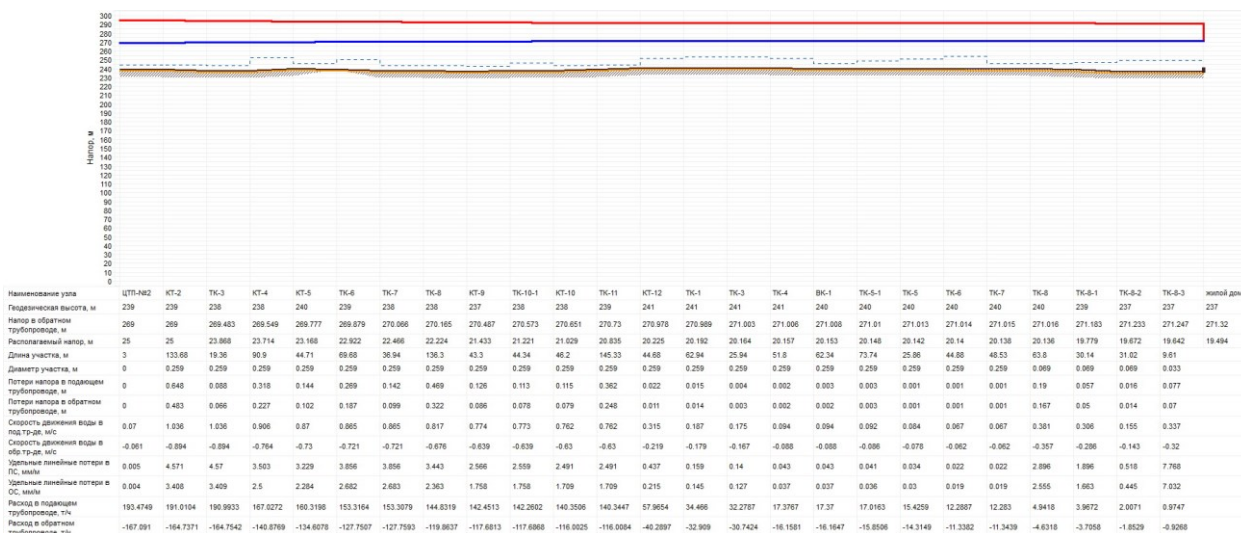
Рисунок 1.9 –Пьезометрический график от ЦТП-2 до жилого дома ул. Октябрьская, 5А
