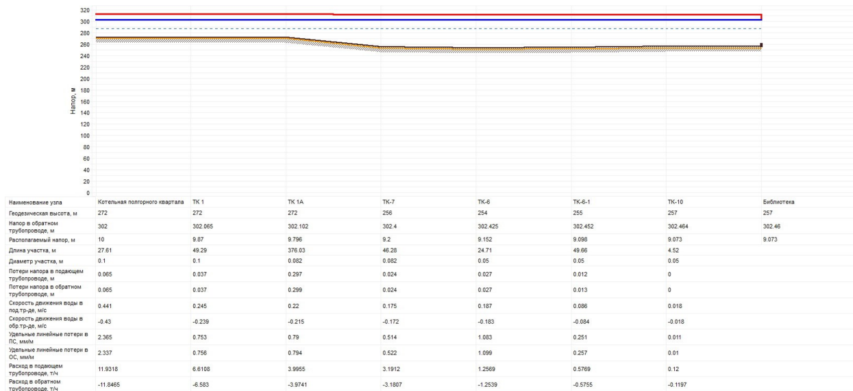
Рисунок 4.11 –Пьезометрический график от Котельной Подгорного квартала до здания Библиотеки
