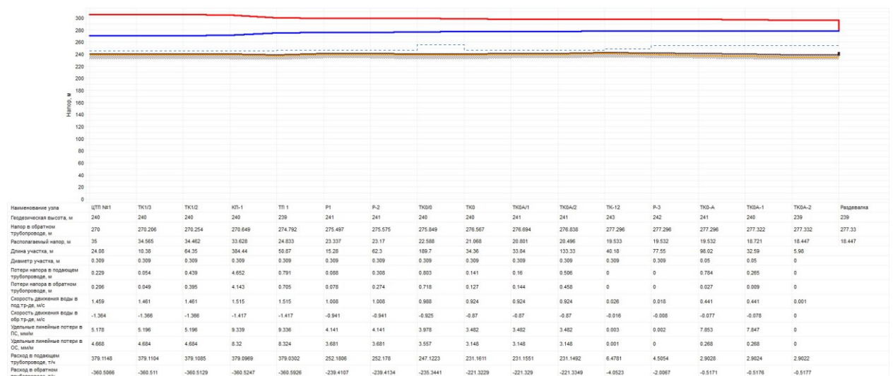
Рисунок 1.6 –Пьезометрический график от ЦТП-1 до здания развальной, МБОУ ДОД "У-АДЮСШ", ул. Гидролизная, 1а
